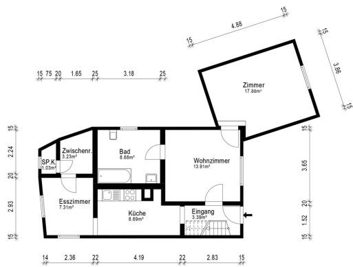
Obergeschoss
