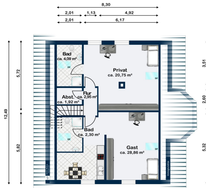
Dachgeschoss
