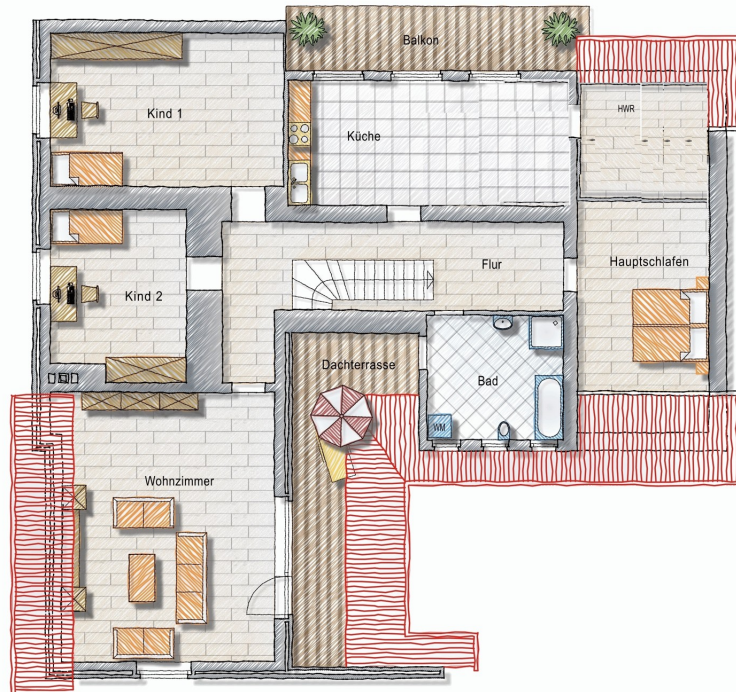
Dachgeschoss
