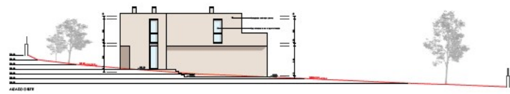
Alzado oeste
