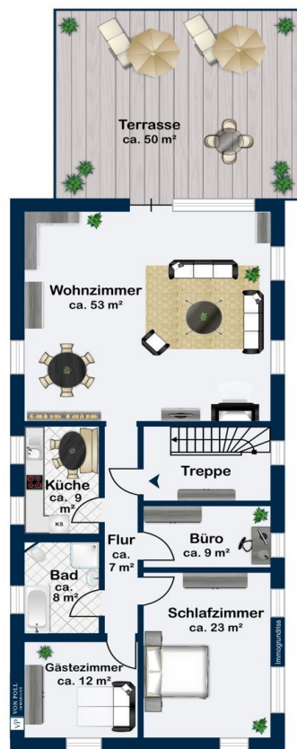
Obergeschoss
