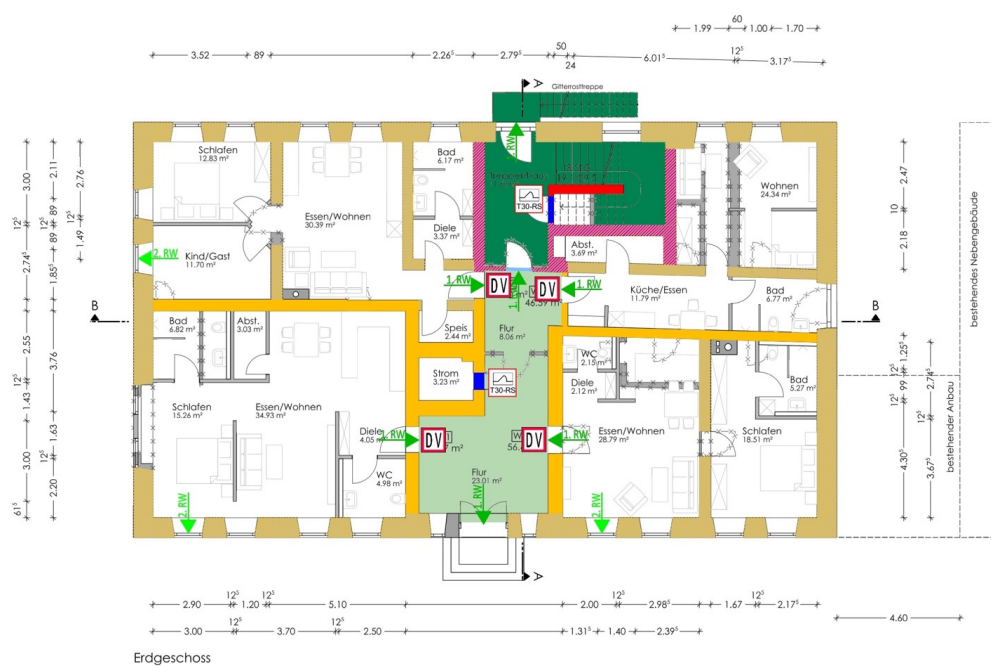
Erdgeschoss
