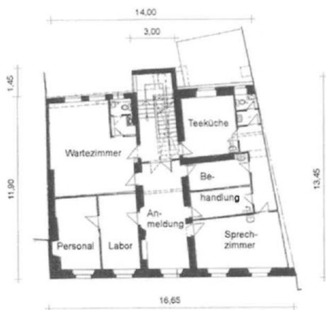
Grundriß Obergeschoß
