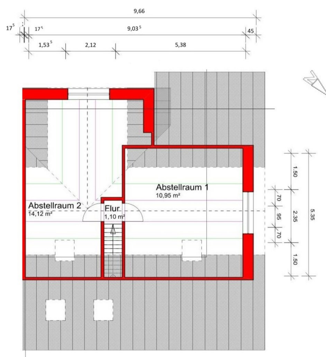
Grundriss Dachgeschoss
