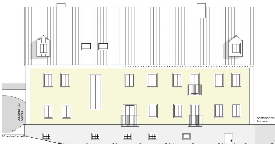
Nordansicht
