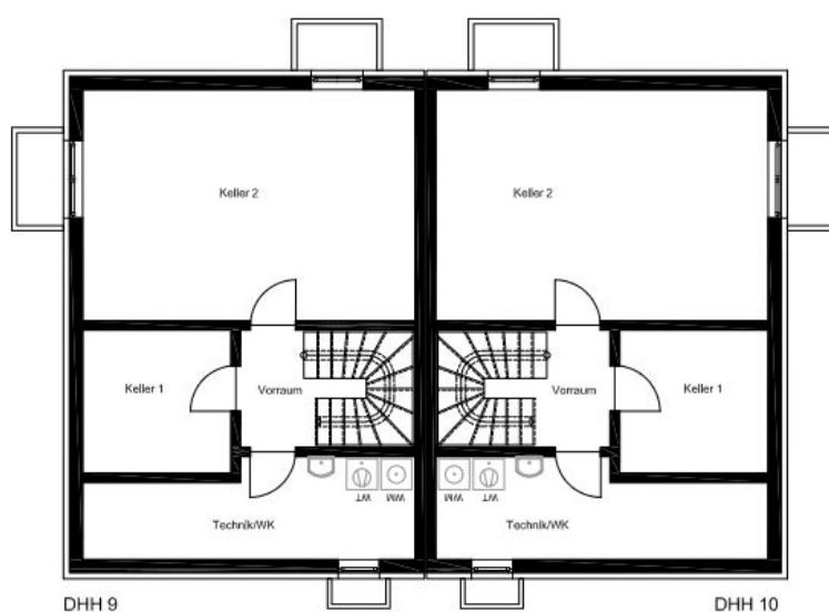
Grundriss UG
