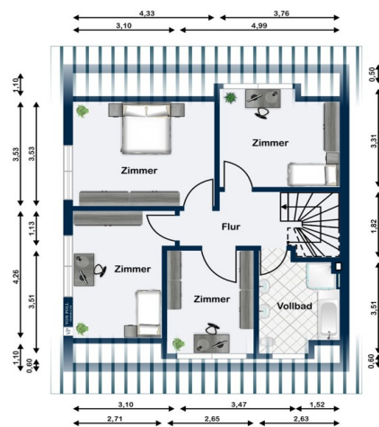
Dachgeschoss
