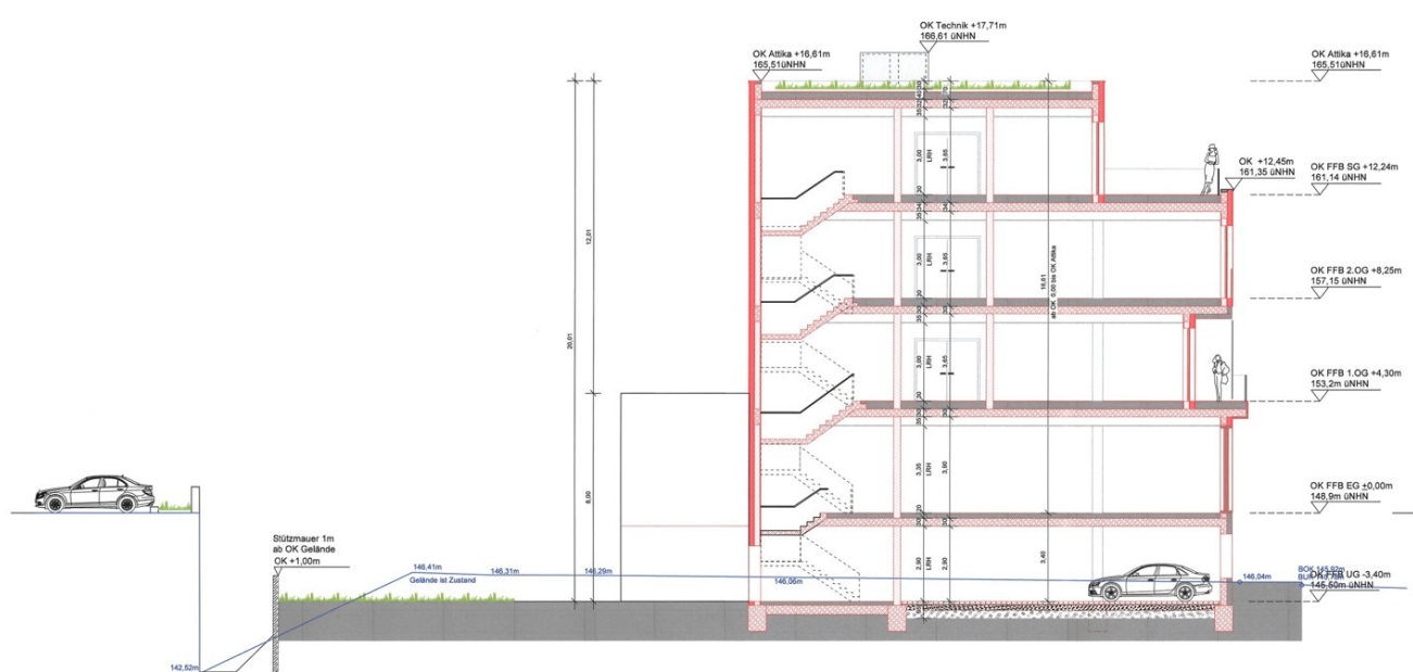
Schnitt B-B
