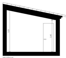
SECCION A-A
